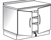
653 (L 70, 80, 90, 100) 2 portes, 2 étagères réglables 2 doors, 2 adjustable shelves
